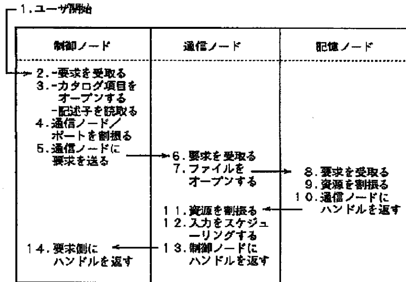
接続用の制御フロー
